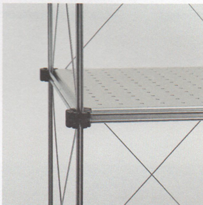
Leitner 6 mattverchromt, Regalablage Aluminium natureloxiert, gelocht.
